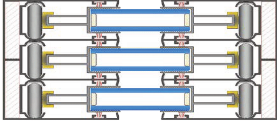
ISICAMLI HAREKETLİ KÜPEŞTE ÜST GÖRÜNÜMÜ THERMOPANE LIFTING BALUSTRADE TOP VIEW
