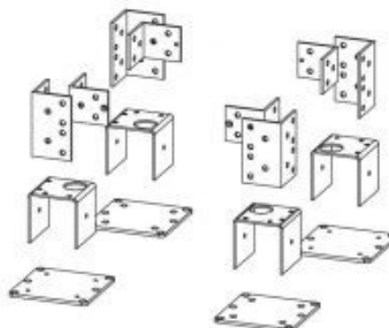
KIT MODULO SINGOLO SINGLE MODULE KIT
