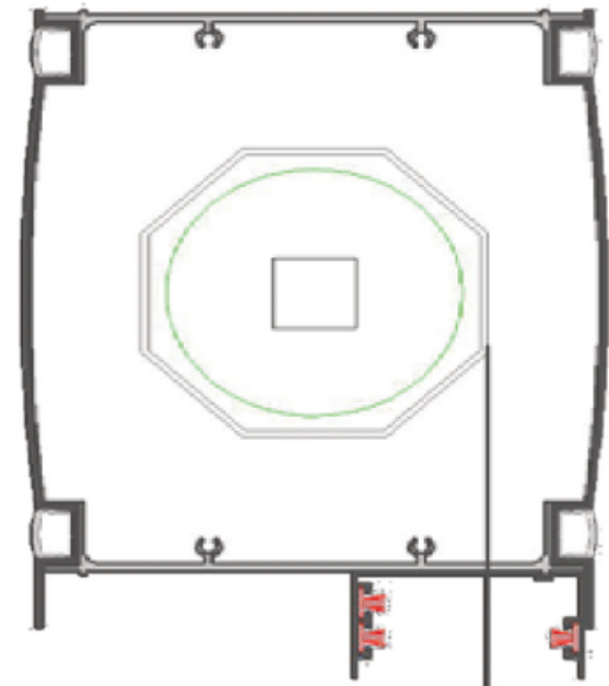
HAREKETLİ KÜPEŞTE AÇIK GÖRÜNÜMÜ LIFTING BALUSTRADE OPEN VIEW
